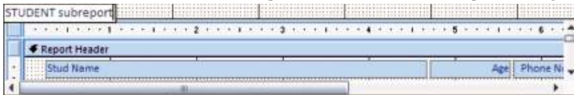
Fig. 2.28: A subreport
